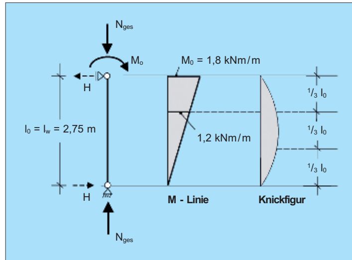
Bild 4.5 b: Momentenverlauf
